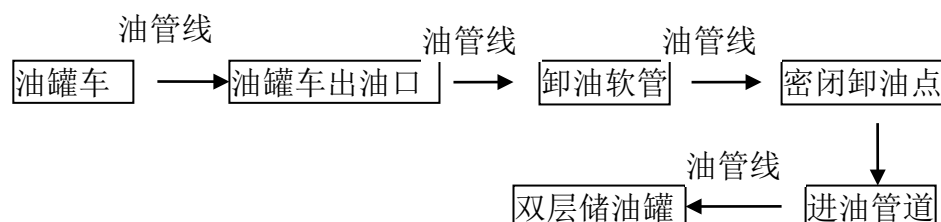
图 2-3 汽油卸油流程框图
